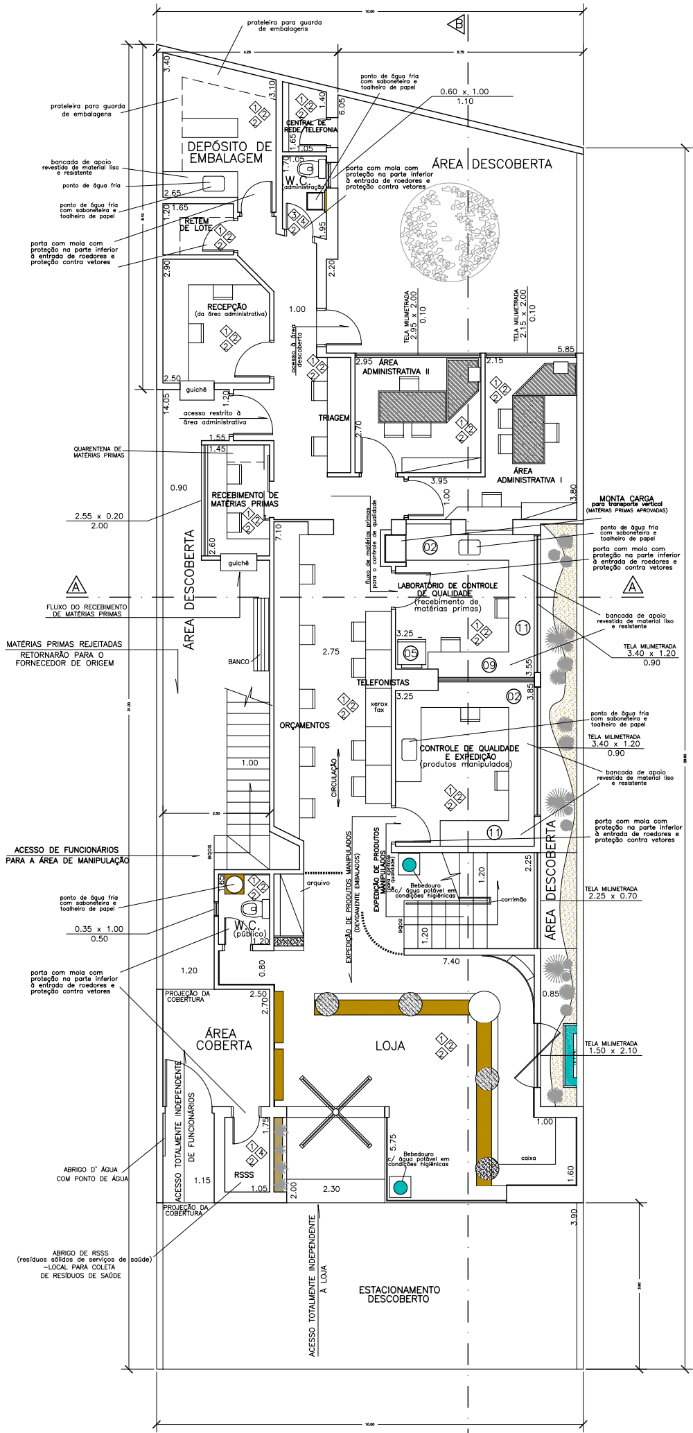
TÉRREO ESCALA 1:100
