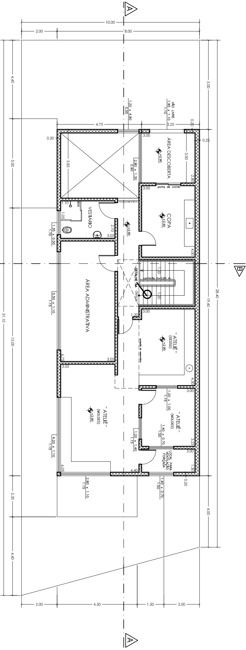
1º PAVIMENTO ESCALA 1:100
